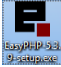
Resim1.36: Kurulum paketi
