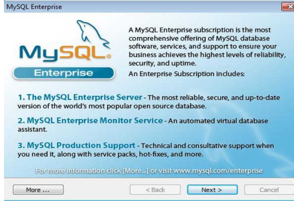
Resim1.25: Bilgilendirme penceresi
