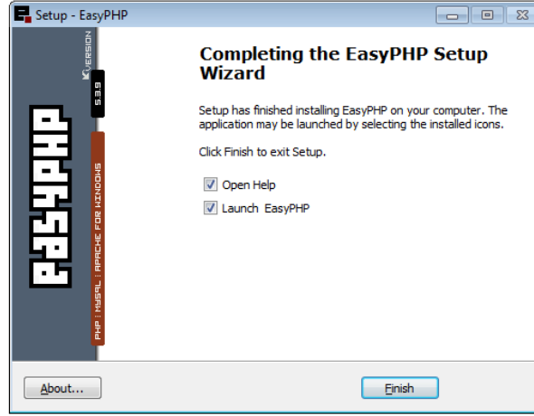
Resim1.43:Kurulumun tamamlanması
