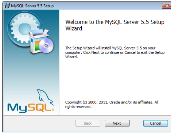
Resim1.20. Kurulumu başlama
