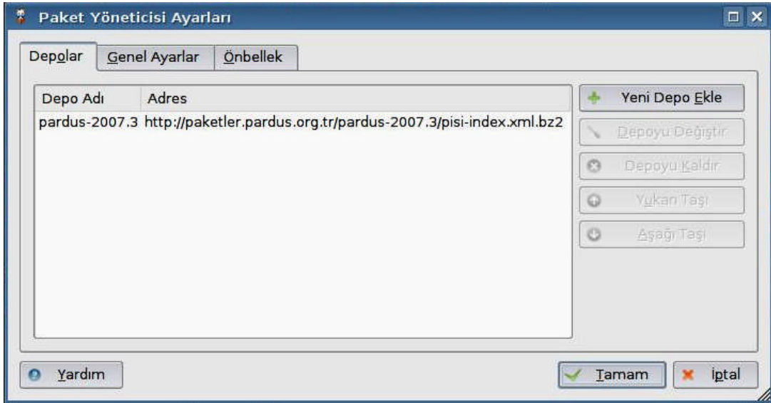
Şekil 3.7: Paket yöneticisi ayarları
