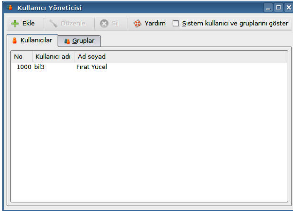
Şekil 1.2: Kullanıcı Yöneticisi
