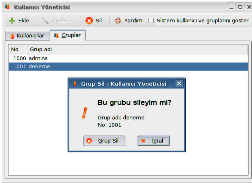
Şekil 1.11: Grup silme
