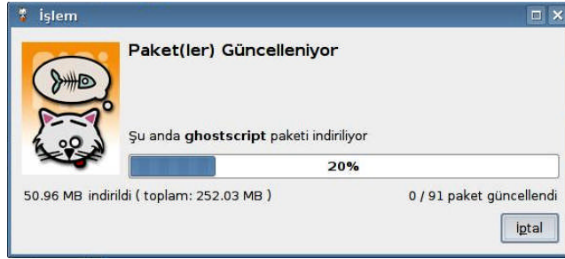
Şekil 3.15: Güncelleme işlemi
