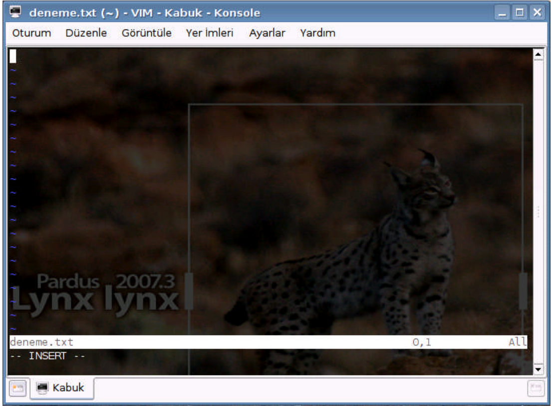
Şekil 2.1: VIM programı
