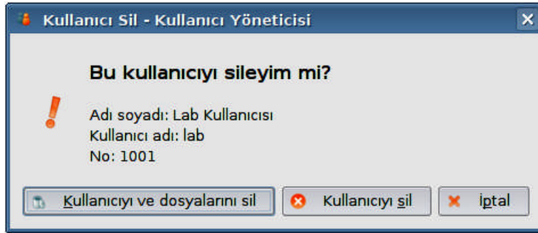
Şekil 1.5. Kullanıcı silme
