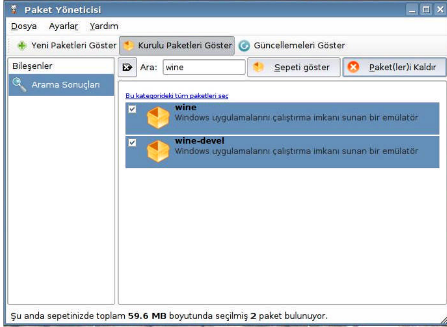
Şekil 3.11: Paket kaldırma
