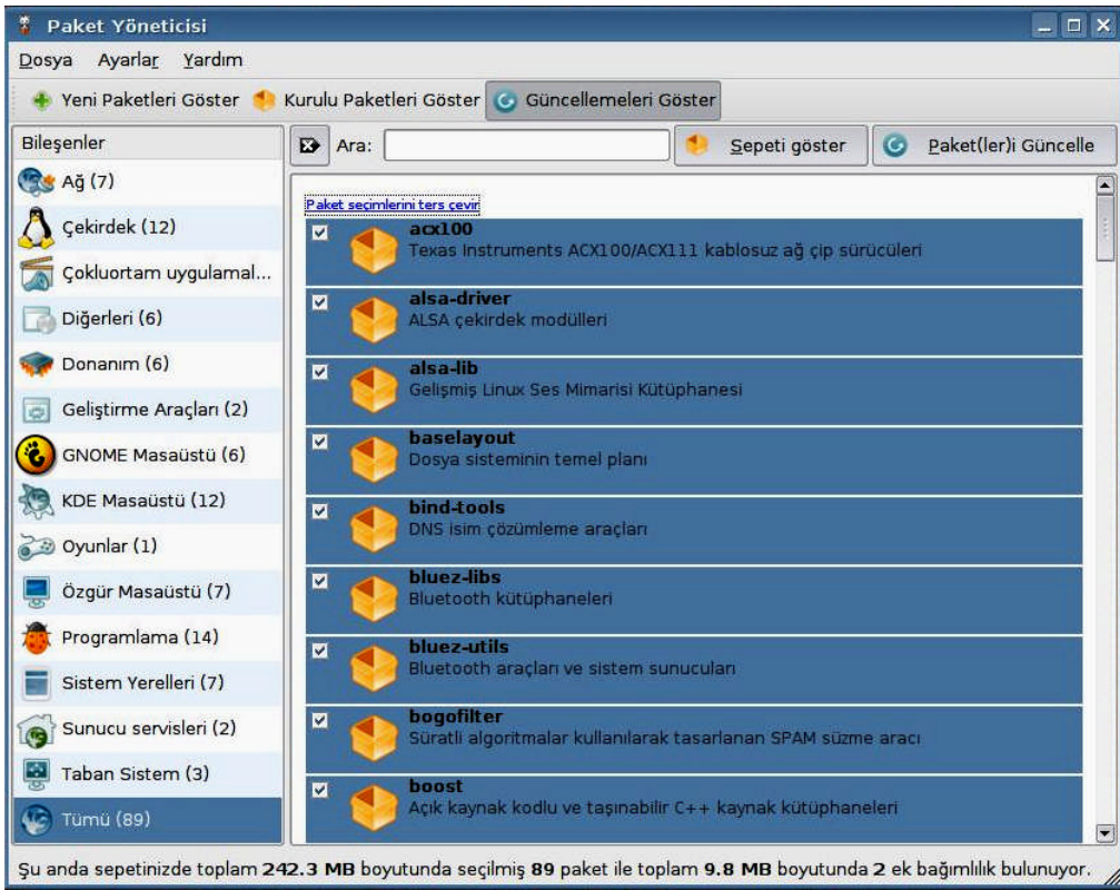
Şekil 3.14: Program güncellemeleri
