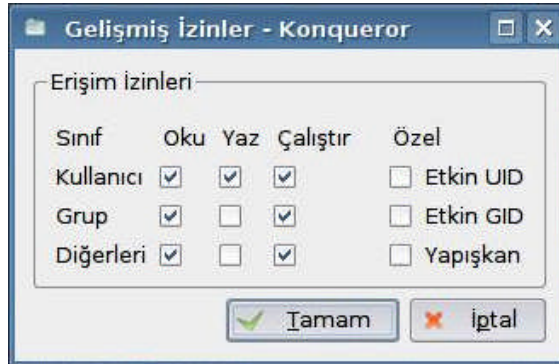
Şekil 1.16 Gelişmiş izinler
