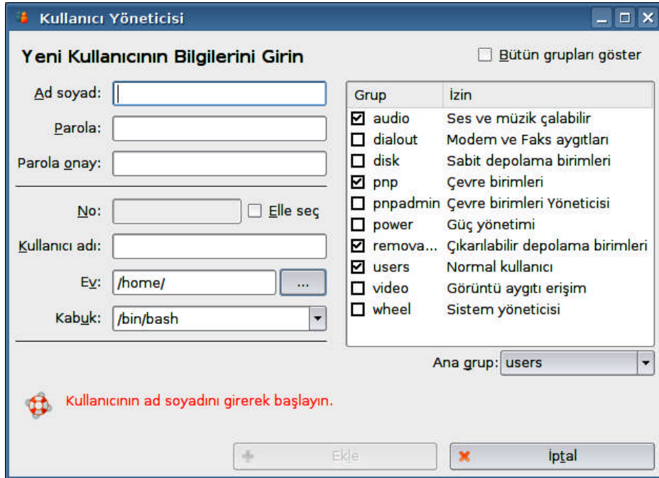
Şekil 1.3: Kullanıcı Yöneticisi
