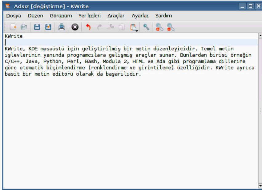
Şekil 2.3: KWrite editörü
