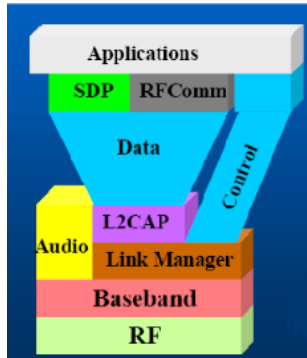
Resim 2.15: Bluetooth teknolojisi protokol kümesi
