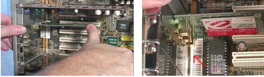
Resim 1.25.:Kablosu ağ adaptörünün takılması
