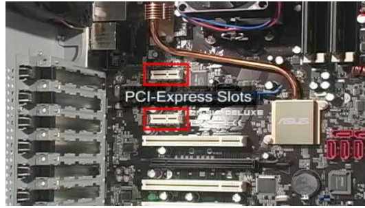
Resim 1.26: PCI-Express slotu
