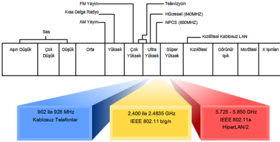
Şekil 1.2: Radyo dalgaları frekans aralığı
