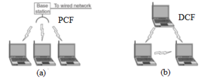
Şekil 2.4: Kablosuz ağ çalışma modları
