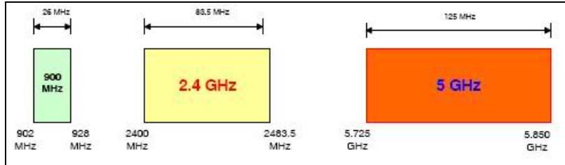
Şekil 1.3.: ISM frekans bantları
