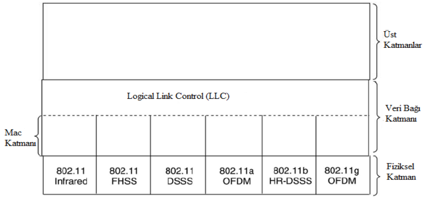
Şekil 2.3: 802.11 protokol yığıtı
