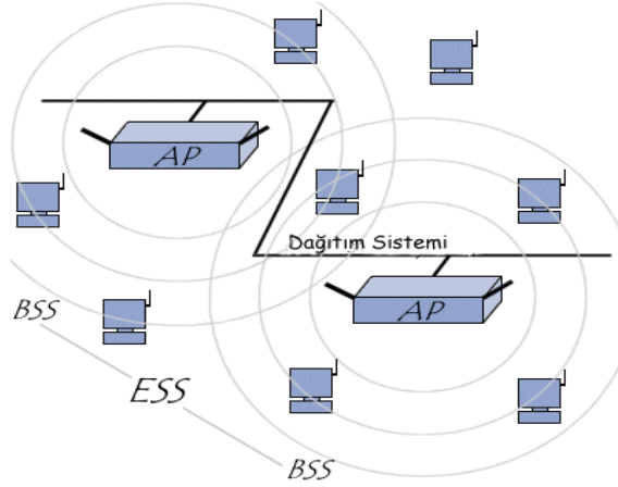
Şekil 1.9: Genişletilmiş servis kümesi (ESS)
