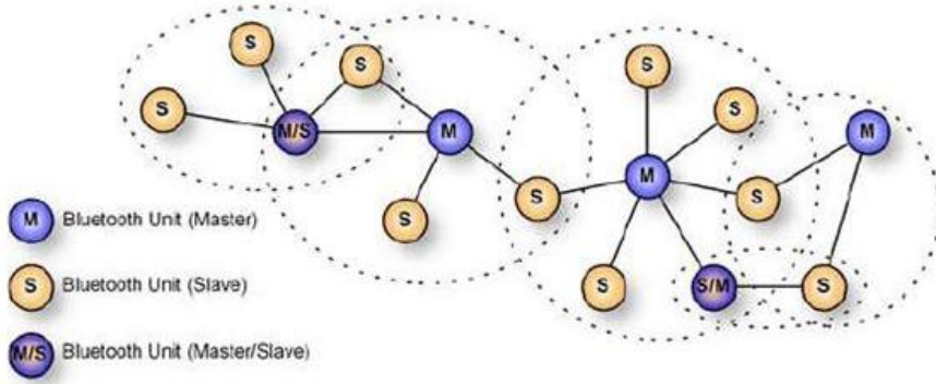
Şekil 2.2: Scatternet topolojisi şematik gösterimi
