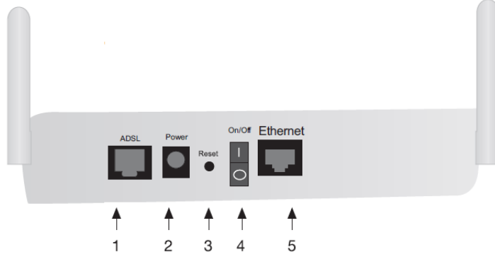
Resim 1.8: Kablosuz modem arkadan görünüş
