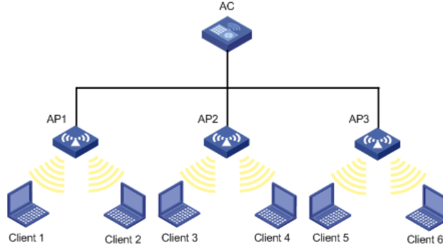
Resim 1.17: Kablosuz LAN'ların erişim noktaları (AP) ile genişletilmesi
