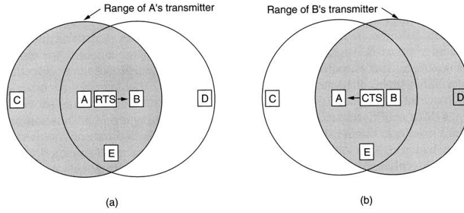
Şekil 2.6: MACA protokolü örneği
