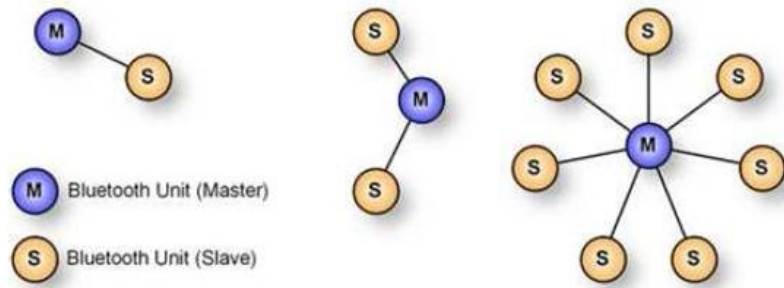
Şekil 2.1: Piconet topolojisi şematik gösterimi
