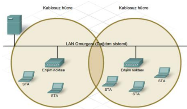
Şekil 1.10: Genişletilmiş servis kümesinde hücre yapısı
